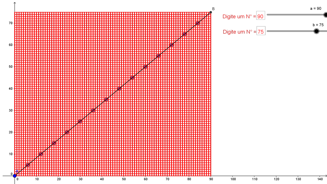
Figura 7: Visualização gráfica- mmc(90, 75) e mdc(90, 75)
